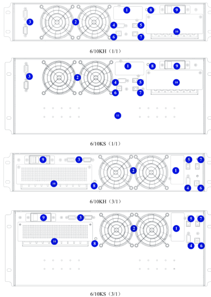
Мал. 2 Задня панель ДБЖ
