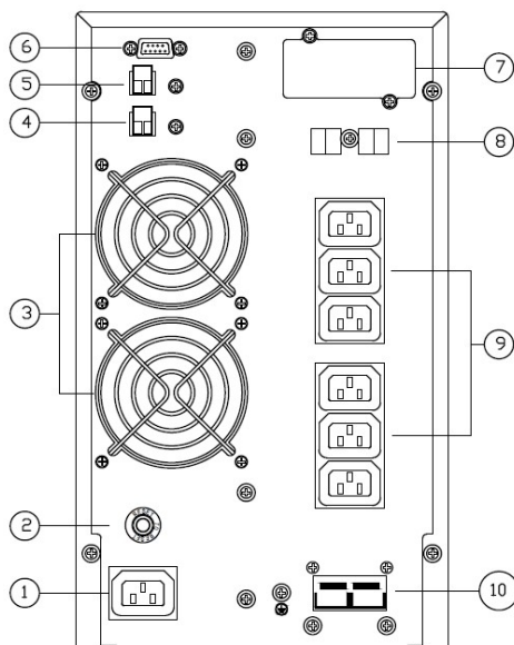
Мал. 3 Задня панель ДБЖ EAST EA900P 3 кВА
