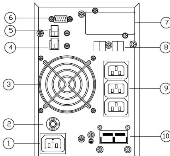
Мал. 2 Задня панель ДБЖ EAST EA900P 1-2 кВА
