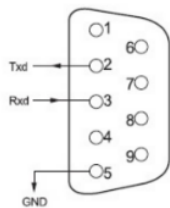
Порт RS232.
