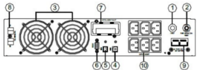
ИБП 2кВа и 3кВА
