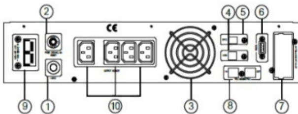
ИБП 1кВА
