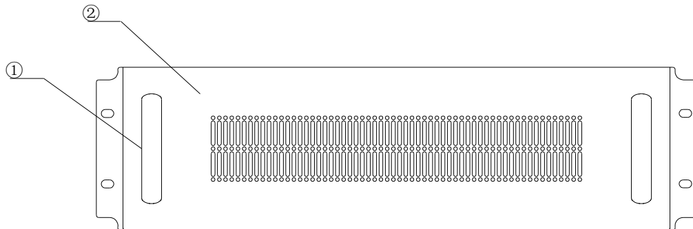
Мал. 3 Передня панель зовнішнього батарейного блоку ДБЖ 6-10 кВА
