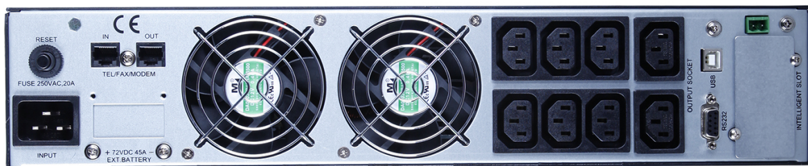
Мал. 2 Задня панель ДБЖ EAST EA900II RT
