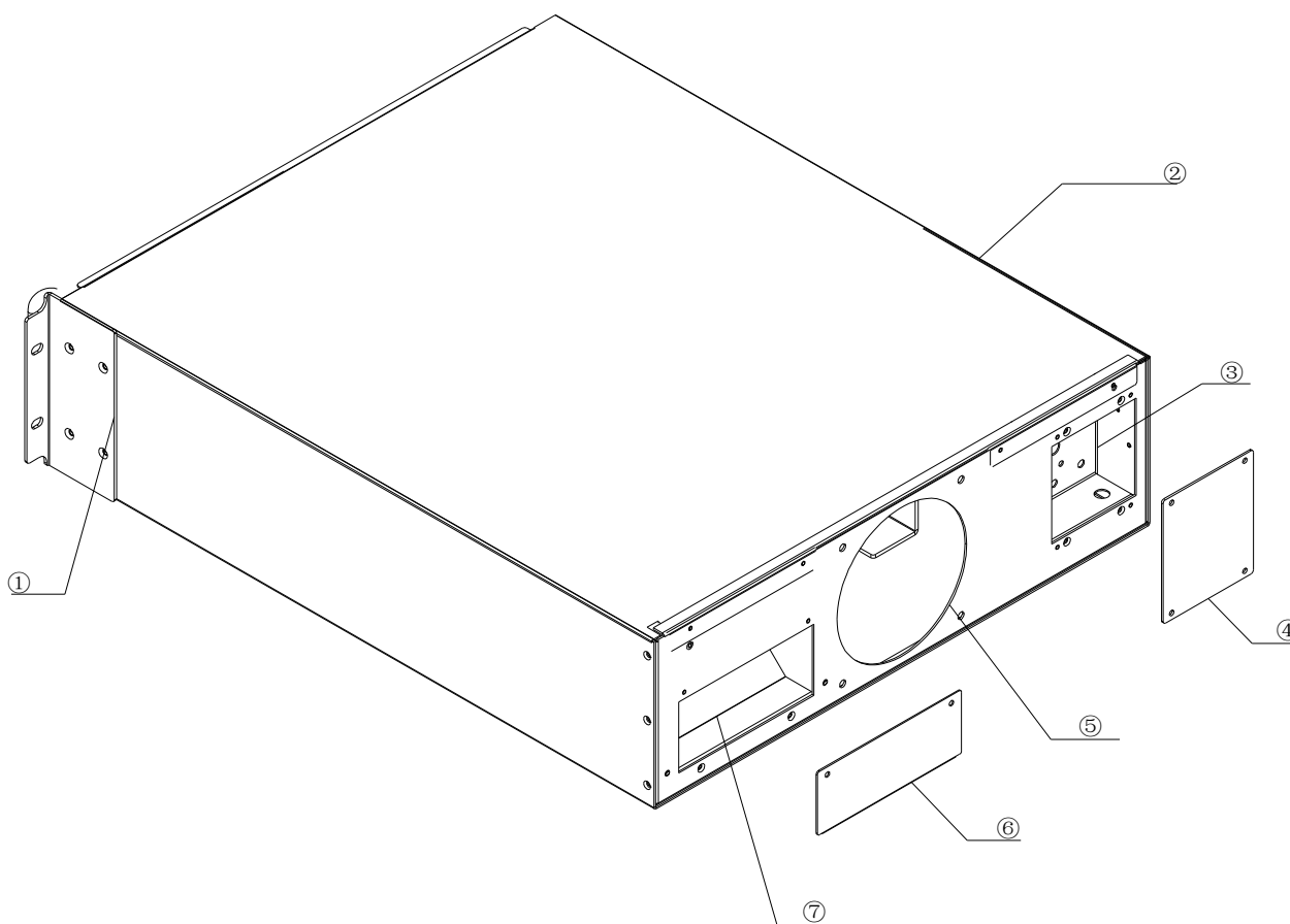
Мал. 4 Задня панель батарейного блоку ДБЖ 6-10 кВА
