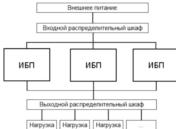
Схема параллельного подключения ДБЖ
